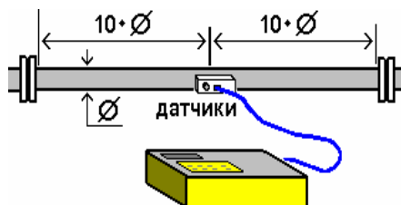
Рис. 10.9. Схема установки датчика для измерения расхода теплоносителя
